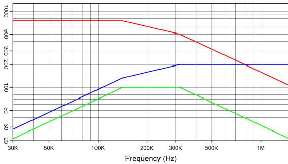
CSM nano 0.2 µF 750 V rms 200 A rms 100 kVA r I(A) — Q(kVA r ) — V rms — V rms
