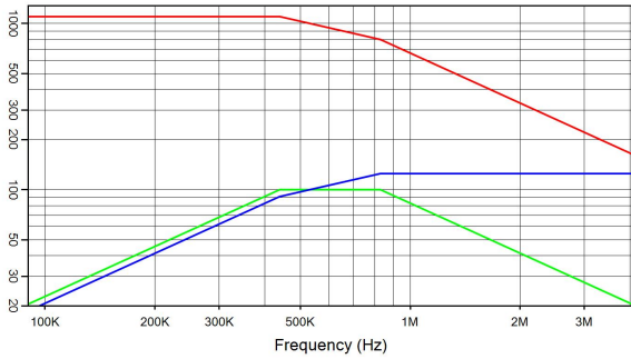
CSM nano 0.03 µF 1100 V rms 125 A rms 100 kVA r I(A) — Q(kVA r ) — V rms — V rms
