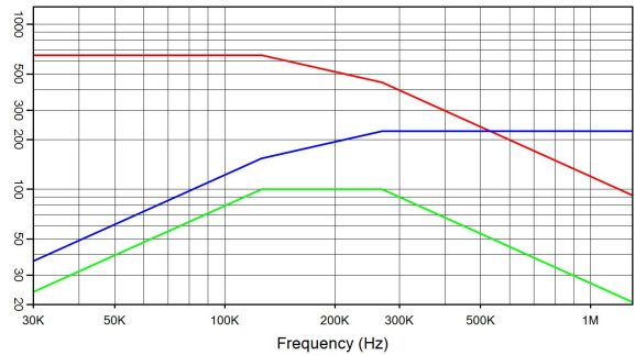
CSM nano 0.3 µF 650 V rms 225 A rms 100 kVA r I(A) — Q(kVA r ) — V rms — V rms
