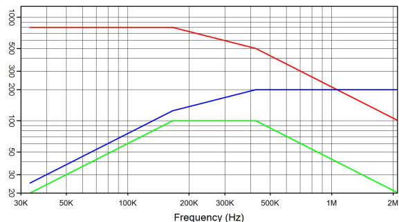
CSM nano 0.15 µF 800 V rms 200 A rms 100 kVA r I(A) — Q(kVA r ) — V rms — V rms
