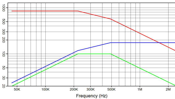
CSM nano 0.1 µF 850 V rms 175 A rms 100 kVA r I(A) — Q(kVA r ) — V rms — V rms
