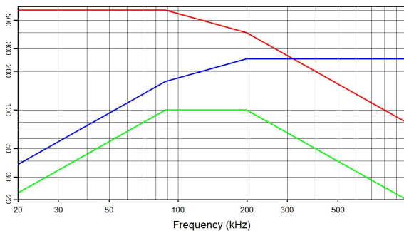
CSM nano 0.5 µF 600 V rms 250 A rms 100 kVA r I(A) — Q(kVA r ) — V rms — V rms
