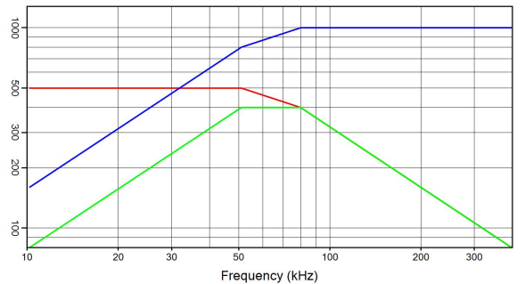
CSP 405A 5 μF 500 V rms 1000 A rms 400 kVA r I(A) — Q(kVA r ) — V rms — V rms
